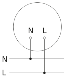
aansluitschema slave/draadloze masterkoppeling
