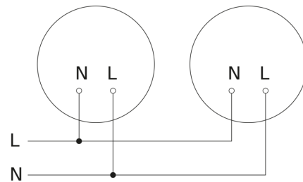
aansluitschema master/master
